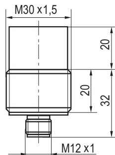
Габаритный чертёж
