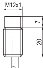
Габаритный чертеж
