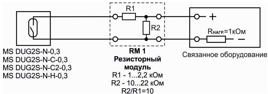
Схема подключения к связанному оборудованию
