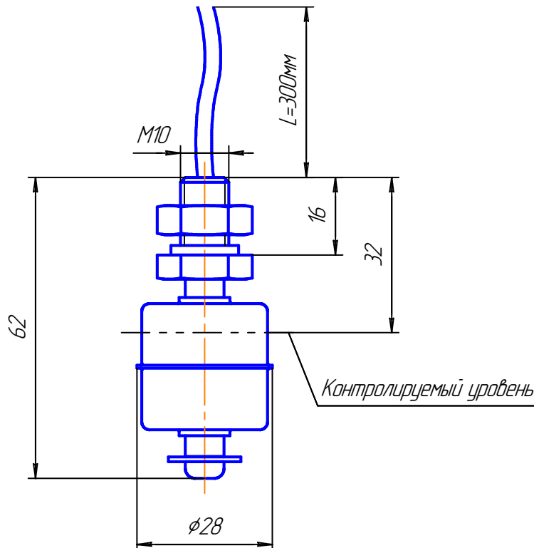
Габаритный чертёж
