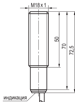
Габаритный чертеж
