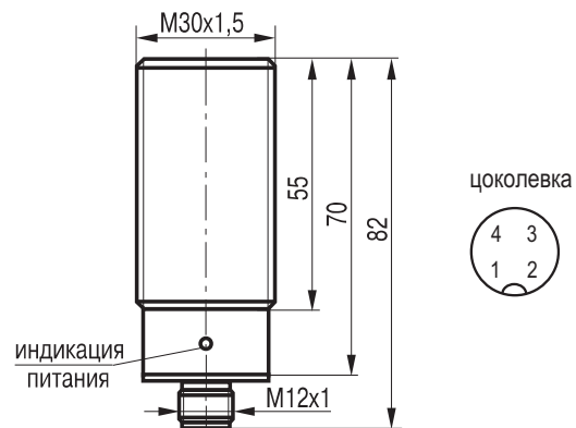
Габаритный чертёж
