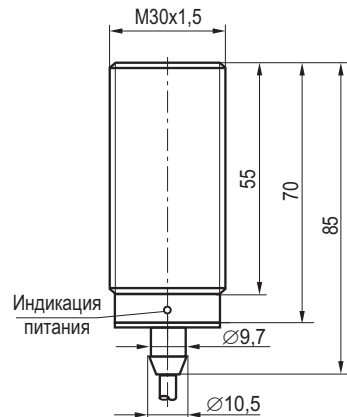
Габаритный чертеж
