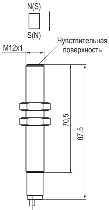
Габаритный чертеж
