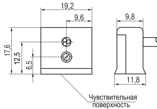
Габаритный чертеж
