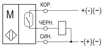
Схема подключения нагрузки
