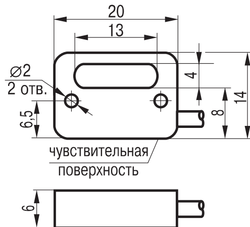
Габаритный чертеж
