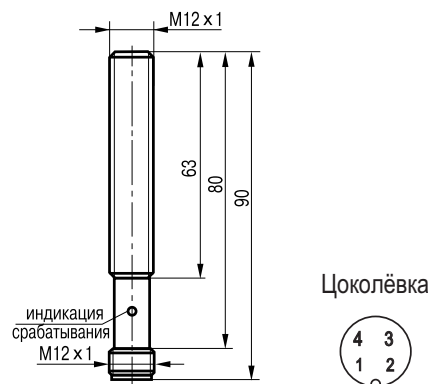
Габаритный чертеж.
