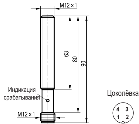
Габаритный чертеж.
