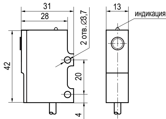
Габаритный чертеж.
