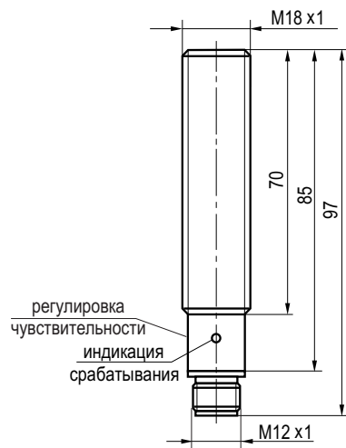
Габаритный чертеж.
