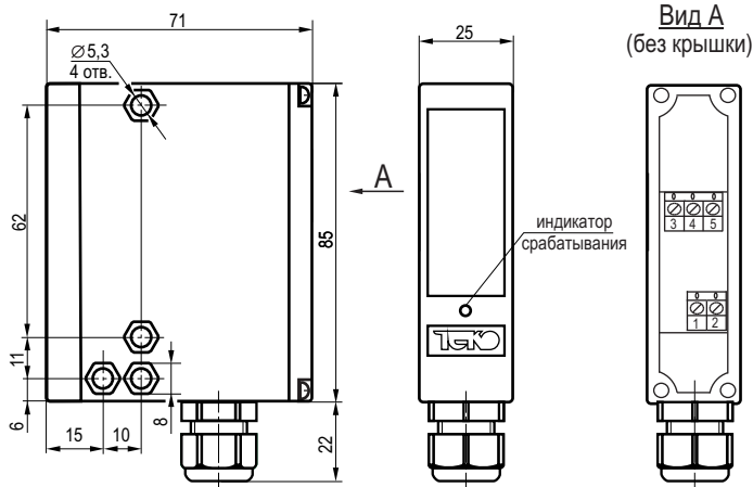
Габаритный чертеж.
