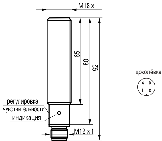
Габаритный чертёж.
