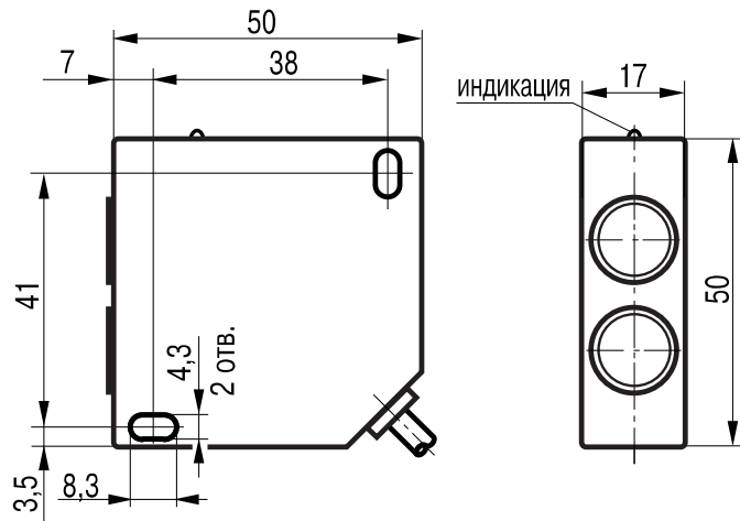
Габаритный чертеж.
