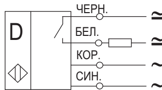
Схема подключения
