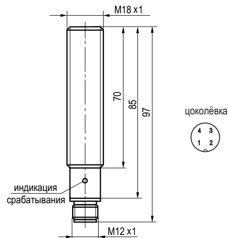
Габаритный чертёж
