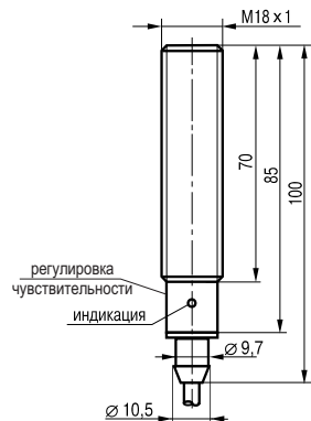
Габаритный чертеж
