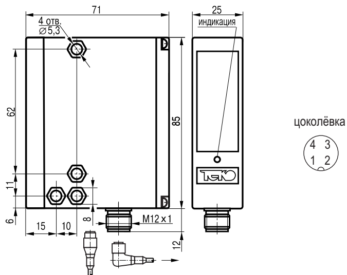
Габаритный чертёж
