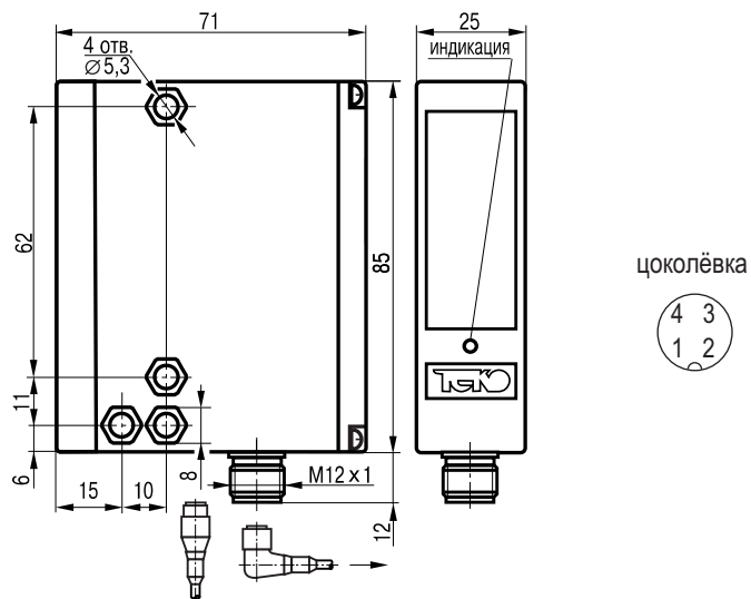
Габаритный чертеж
