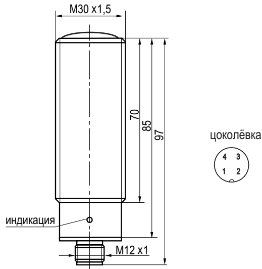
Габаритный чертёж
