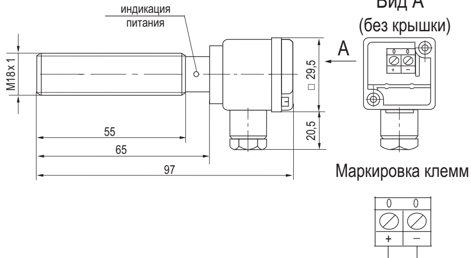
Габаритный чертеж
