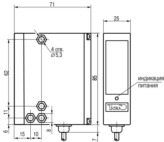
Габаритный чертеж
