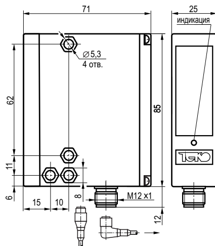
Габаритный чертеж
