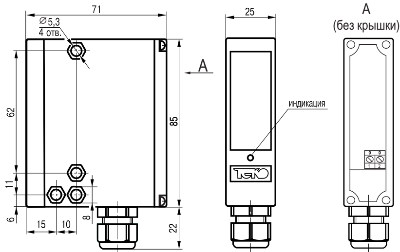
Габаритный чертеж
