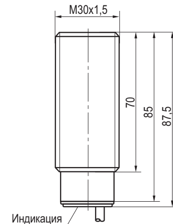
Габаритный чертёж
