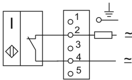
Схема подключения активной нагрузки
