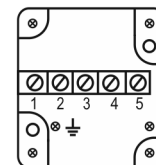
Вид на клеммную коробку (без крышки)
