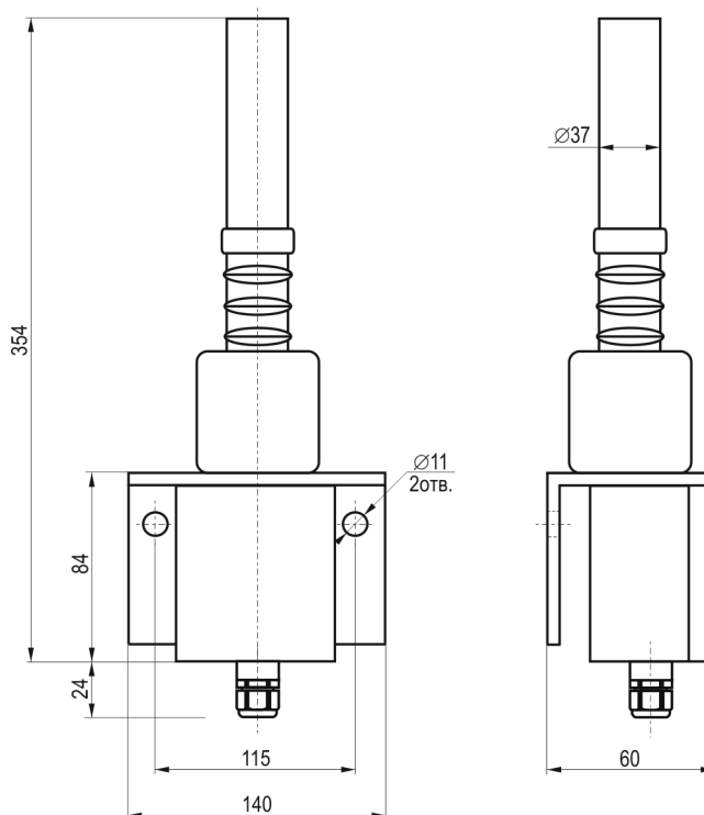
Габаритный чертеж
