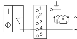
Схемы подключения индуктивной нагрузки
