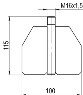
Удлинитель - Лопатка №1
