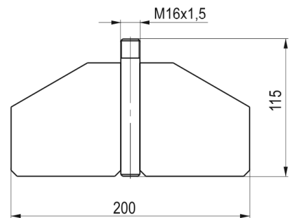
Удлинитель - Лопатка №2
