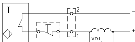
Схема подключения индуктивной нагрузки
