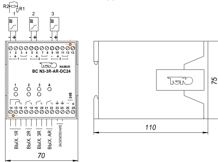
ГАБАРИТНЫЙ ЧЕРТЕЖ СХЕМА ПОДКЛЮЧЕНИЯ
