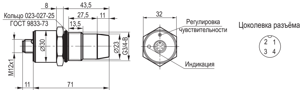
Габаритный чертёж
