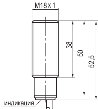
Габаритный чертёж
