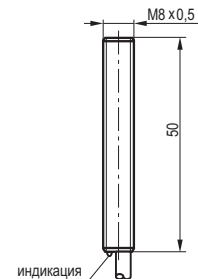
Габаритный чертёж
