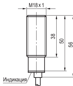
Габаритный чертеж
