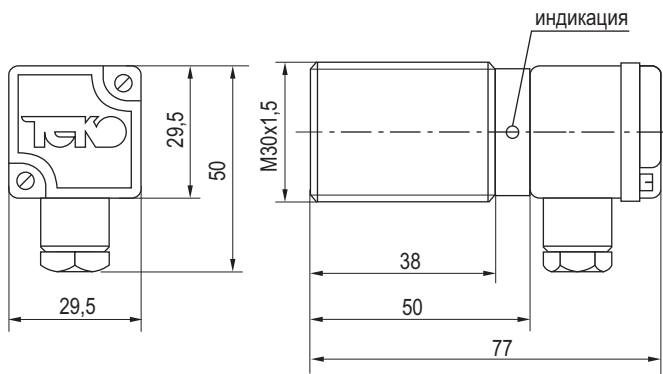
Габаритный чертеж
