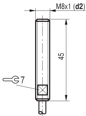
Габаритный чертеж
