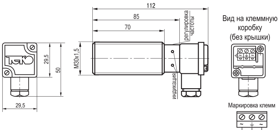
Габаритный чертеж
