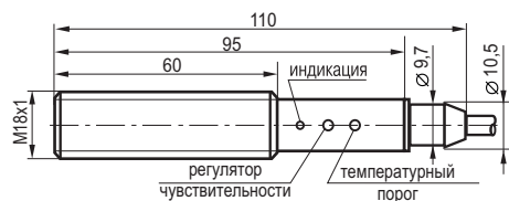
Габаритный чертёж.
