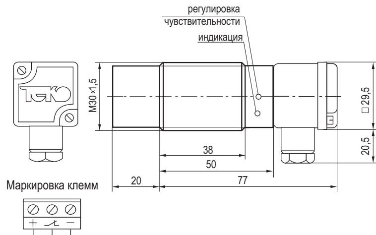
Габаритный чертеж
