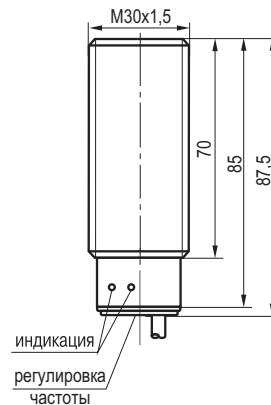
Габаритный чертёж
