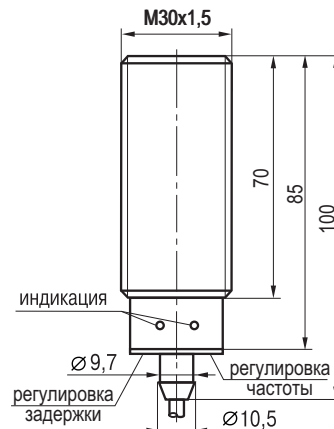
Габаритный чертеж
