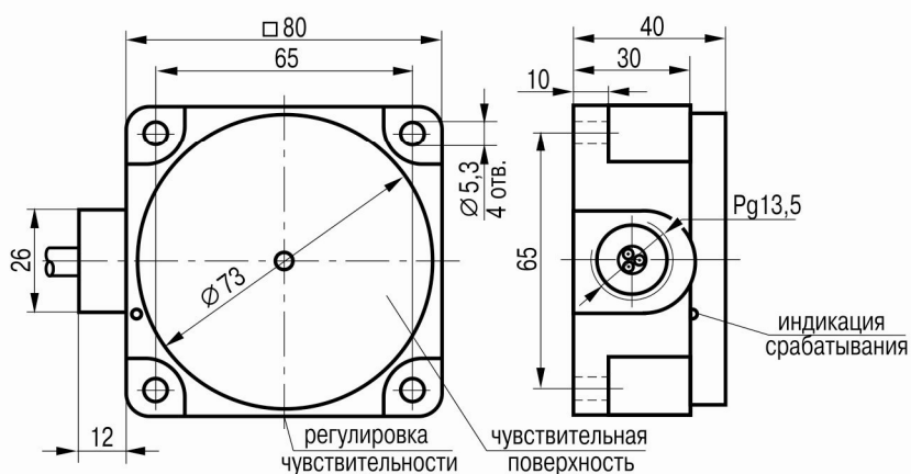
Габаритный чертёж
